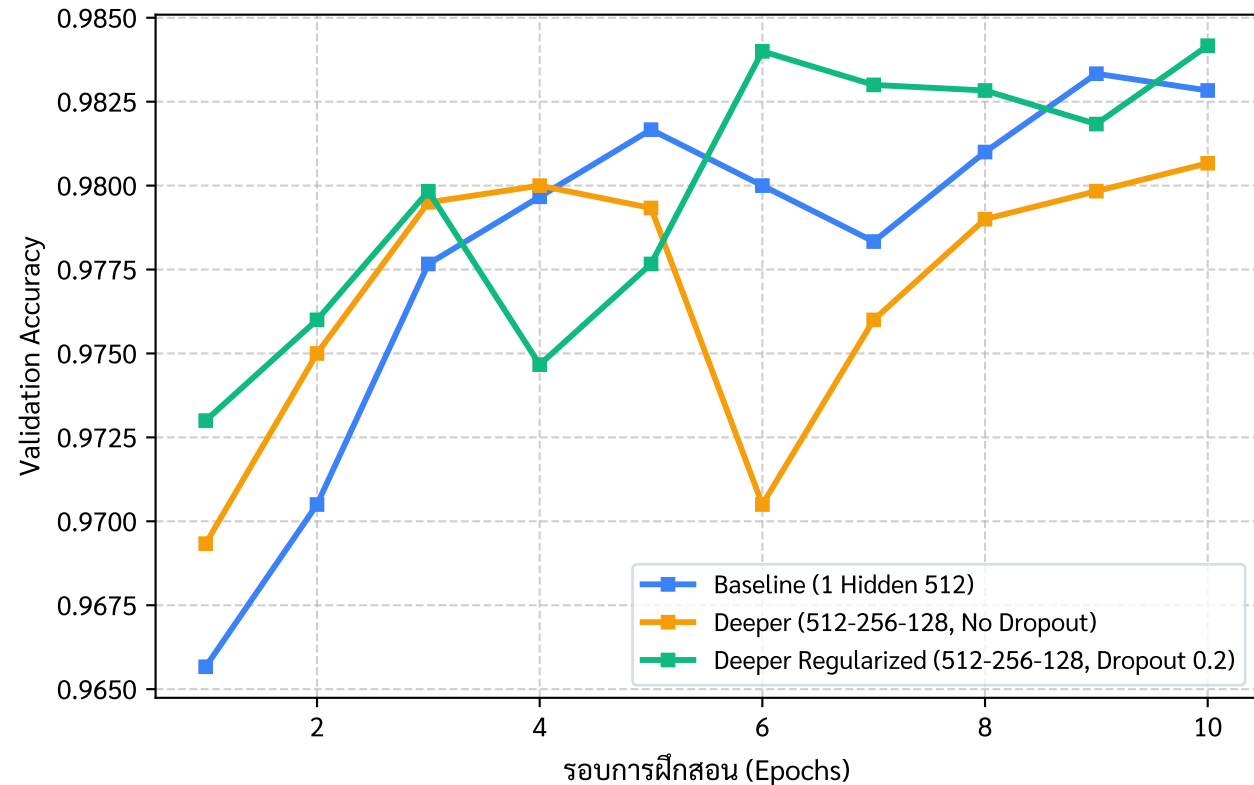
Validation Accuracy เปรียบเทียบตามสถาปัตยกรรม
