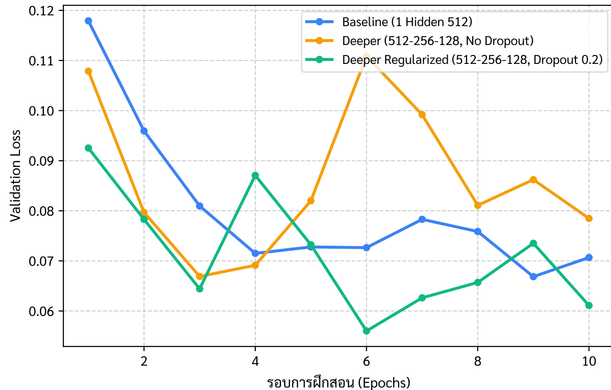
Validation Loss เปรียบเทียบตามสถาปัตยกรรม
